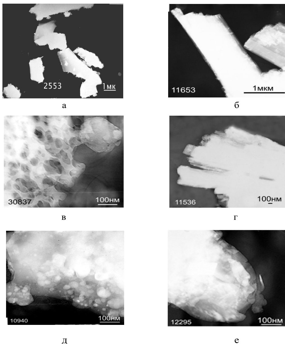
Рис.5. Электронно-микроскопические снимки частиц кварца и волластонита в исходном состоянии (а, б), после УЗО в воде (в, г) и в 10% растворе мочевины (\text{NH}_2)_2\text{CO} в воде (д, е) [23]
