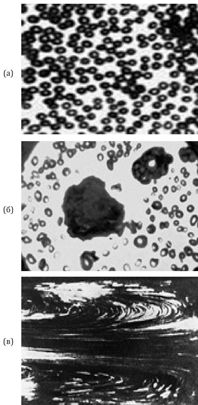
Рис.2. Кавитационные пузырьки (а), схлопывание (б) и потоки (в), возникающие в рабочей жидкости при схлопывании кавитационных полостей в процессе ультразвуковой обработки жидкости [15]
