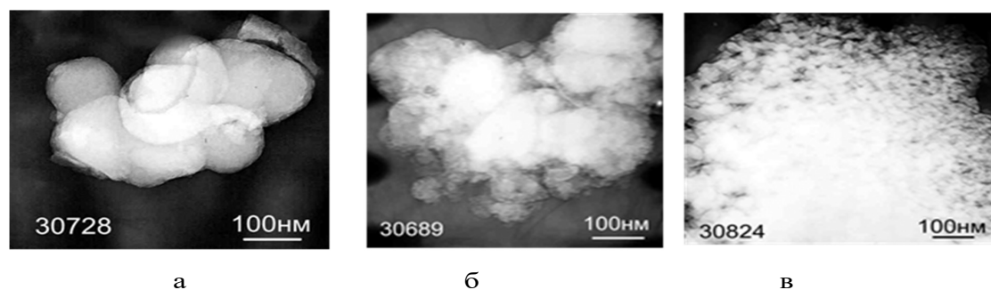
Рис. 6. Электронно - микроскопические снимки частиц диоксида кремния после МХО в шаровой мельнице в водном растворе этилового спирта (а) и глицерина (б) и после УЗО (в) в водном растворе этилового спирта [33]
