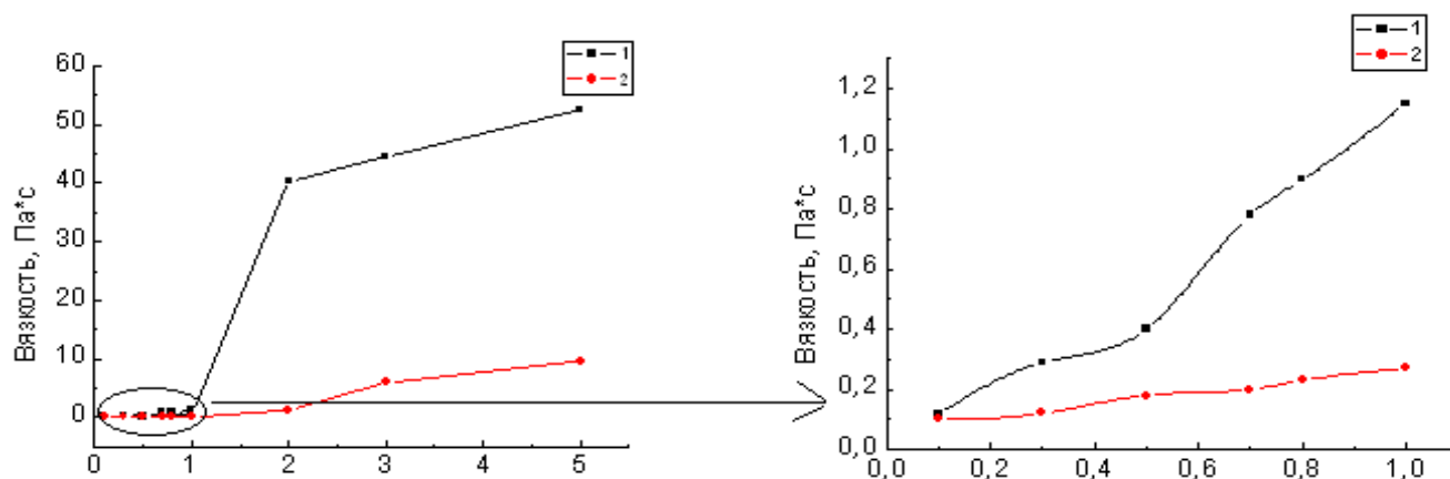
Рис. 7. Изменение вязкости гелевой системы от содержания эфира целлюлозы в водно-глицериновых растворах до (1) и после УЗ обработки (2) [33]
