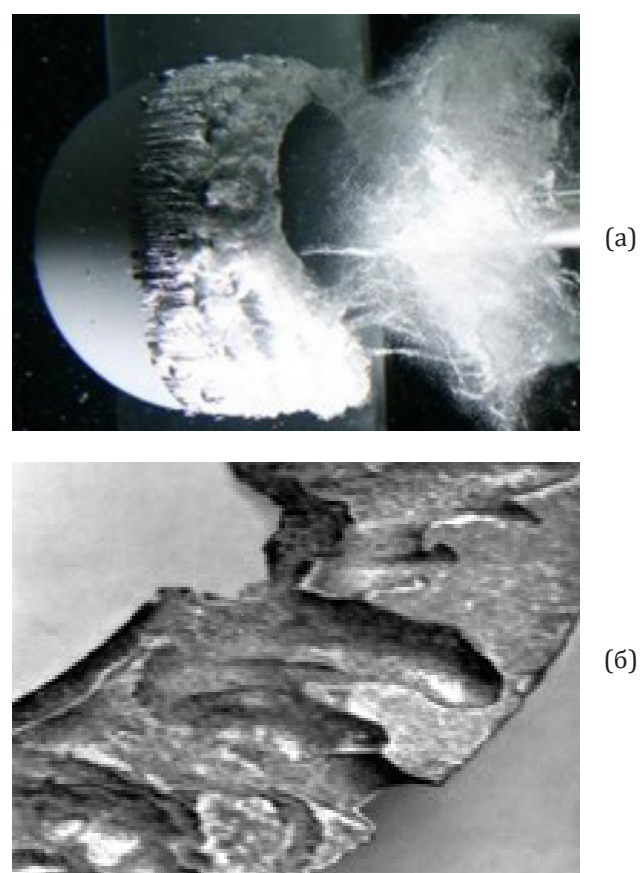
Рис. 3. Эффект схлопывания кавитационных пузырьков (а) и механическая эрозия поверхности материалов (б), при ультразвуковой обработке системы [17]
