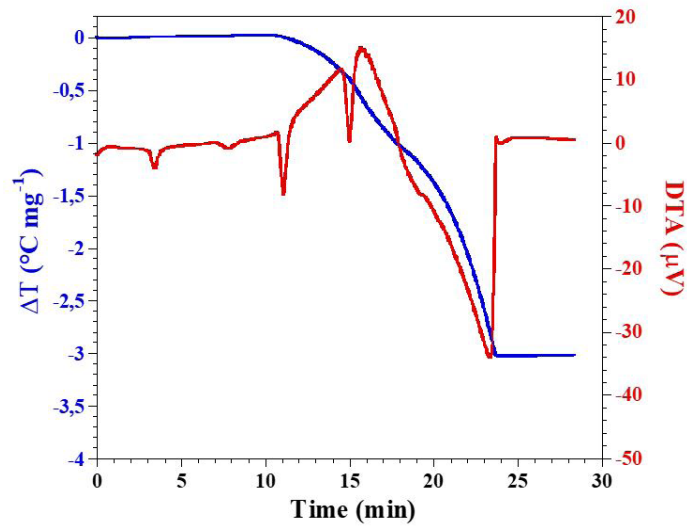
Рис. 4. ДТА-ТГ термического разложения \text{NH}_4\text{NO}_3 с добавкой КМЦ
