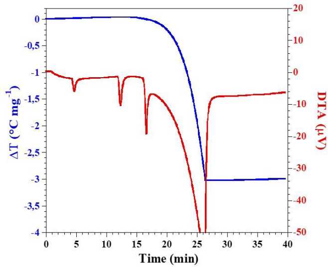
Рис. 3. ДТА-ТГ термического разложения \text{NH}_4\text{NO}_3 в чистом виде
