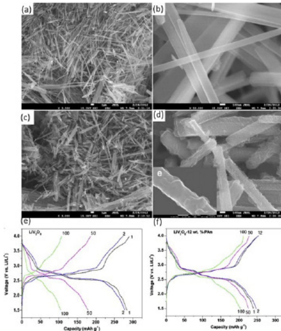
Рис. 2. (a, b) СЭМ-изображения чистого \text{LiV}_3\text{O}_8 и (c, d) \text{LiV}_3\text{O}_8 -12% PANi-композиата (e) Кривые заряда-разряда для \text{LiV}_3\text{O}_8 и (f) \text{LiV}_3\text{O}_8 - 12% композиата PANi [34]
